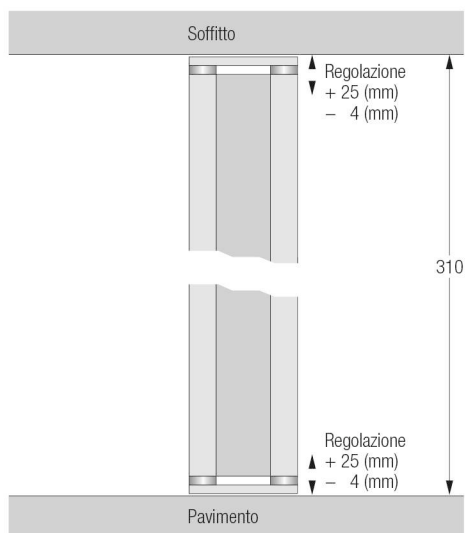
Montante pavimento/soffitto
