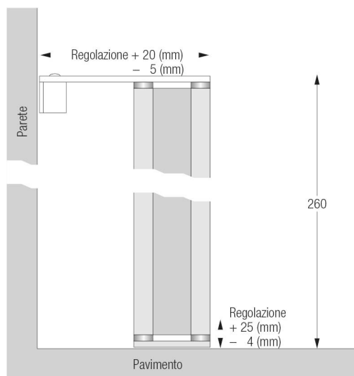
Montante pavimento/parete
