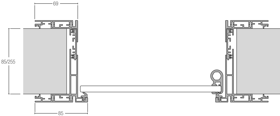
Stipite Light versione a tirare. Light frame pull option.
