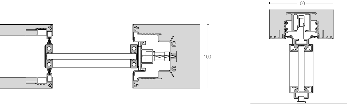
Predisposizione per cassonetto Scrigno® Essential. Arrangement for Scrigno metal box® Essential.
