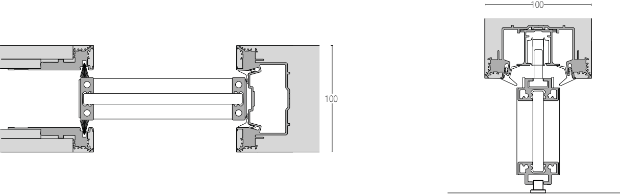
Predisposizione per cassonetto Eclisse® Syntesis. Arrangement for Eclisse metal box® Syntesis.
