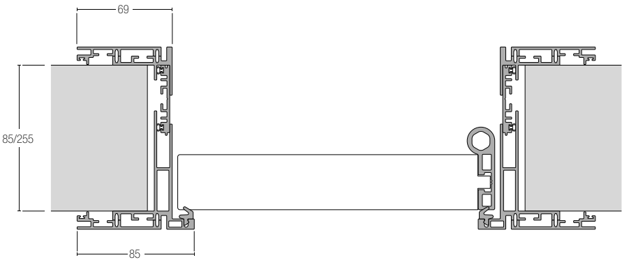
Stipite Light versione a spingere. Light frame push option.
